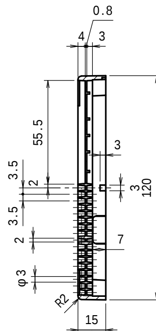
A-A断面図
